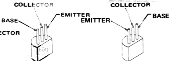
2SC458B (Q1016)
